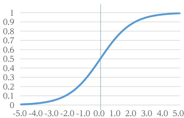
図 1 標準シグモイド関数のイメージ
